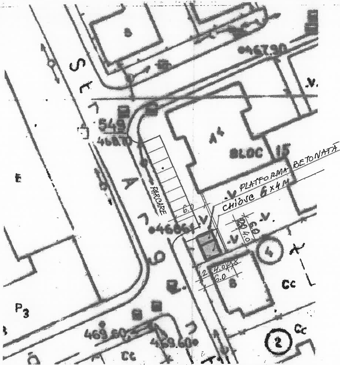
PLAN AMPLASAMENT SC. 1:500
